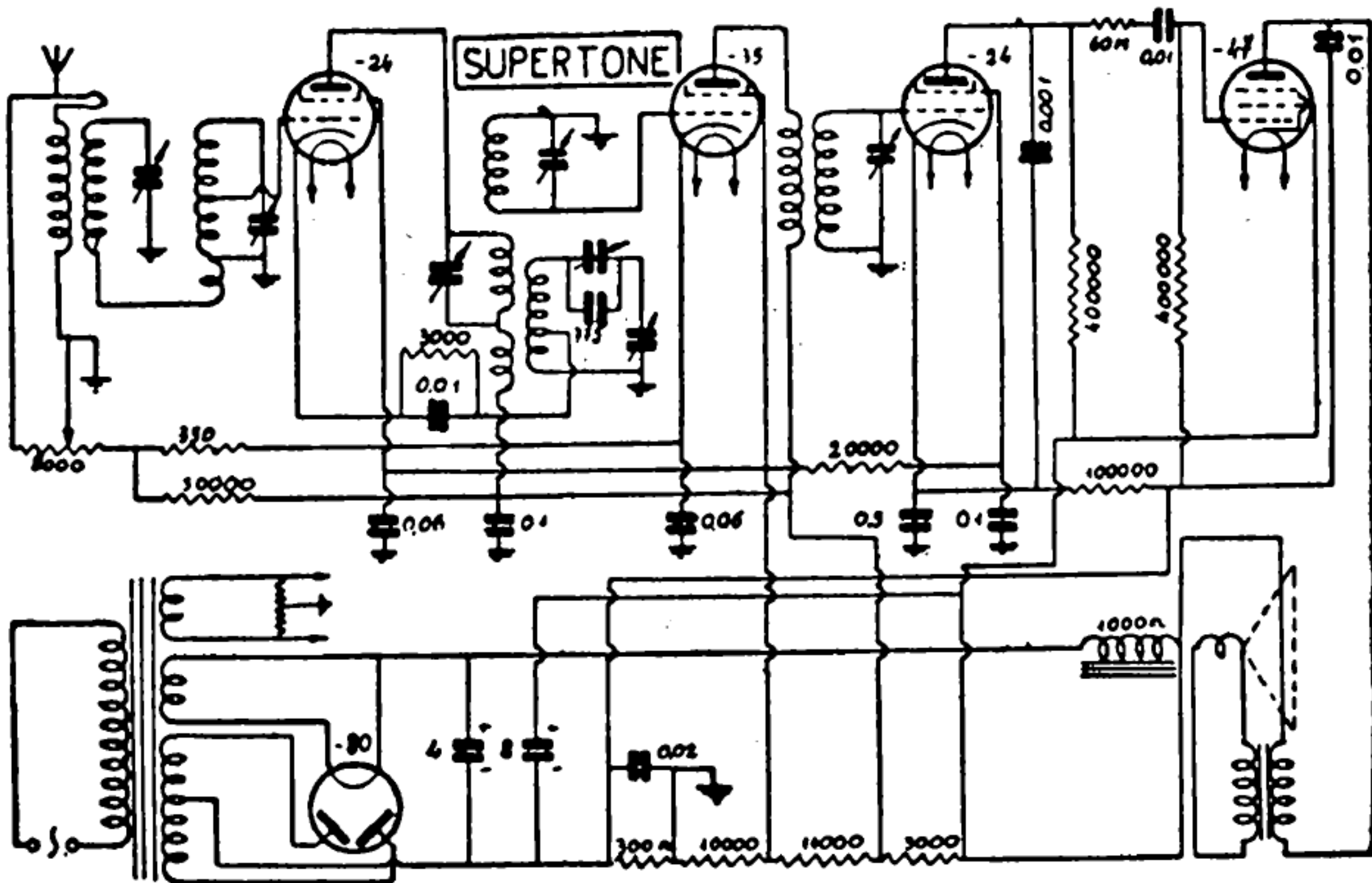
SUPERTONE RADIO. — Mod. 480. — Valvole e valori indicati nello schema. — MF: 175 kHz. — Produz. 1932.
